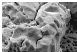
扭矩测试: REM 中脆性劣质材料的折断图。
